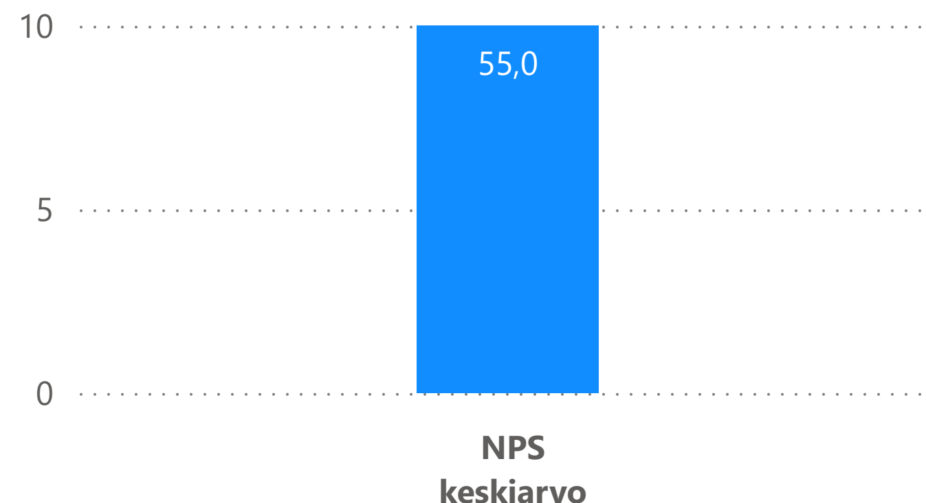
NPS keskiarvo (-100 - +100)
